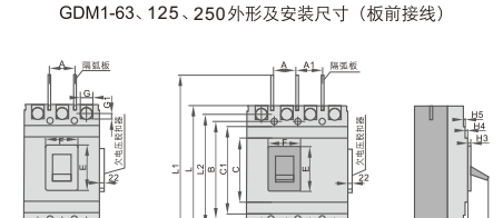
GDM1-63、125、250外形及安装尺寸(板前接线)
